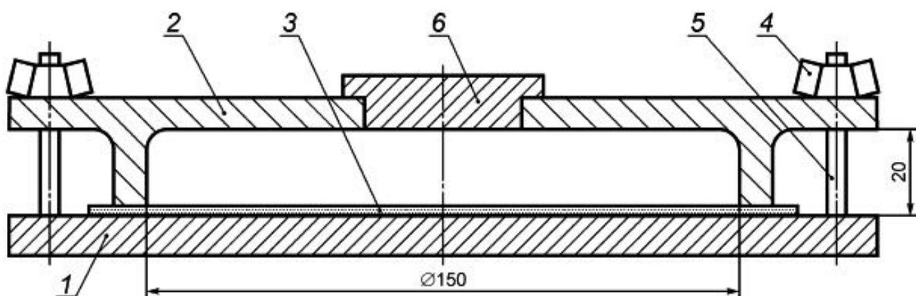
Рисунок У.1 - Устройство для испытания полимерных вставок в контакте с инъекционно-уплотняющим составом
