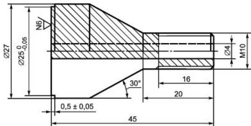
Рисунок М.2 - Конический штамп
