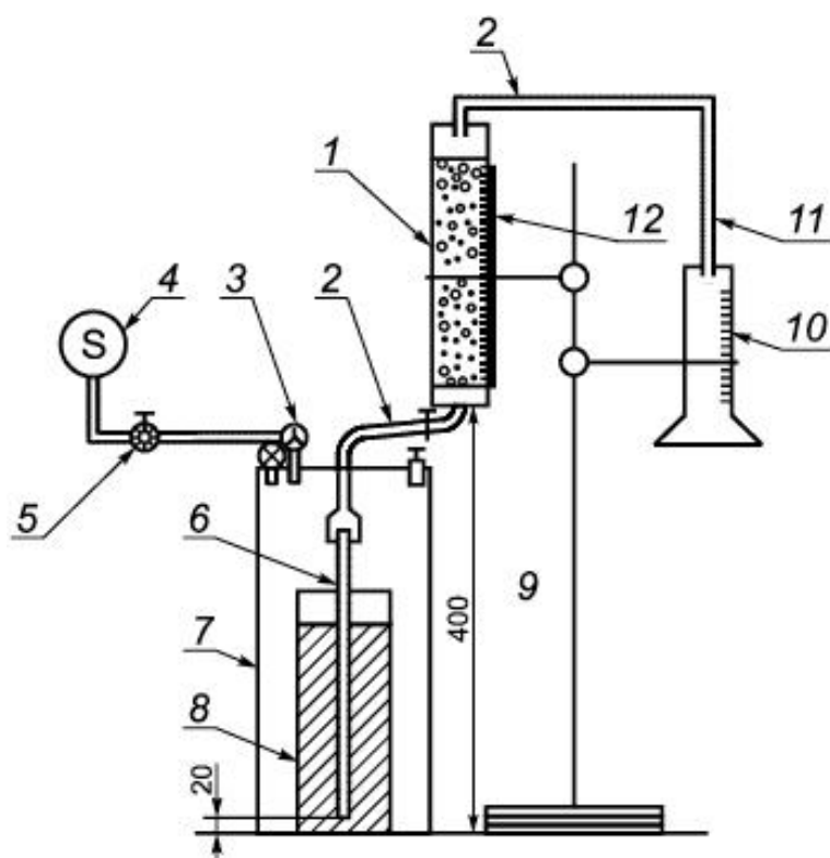
Рисунок Л.1 - Схема установки и испытаний нагнетаемости инъекционно-уплотнительных составов в песчаную колонку
