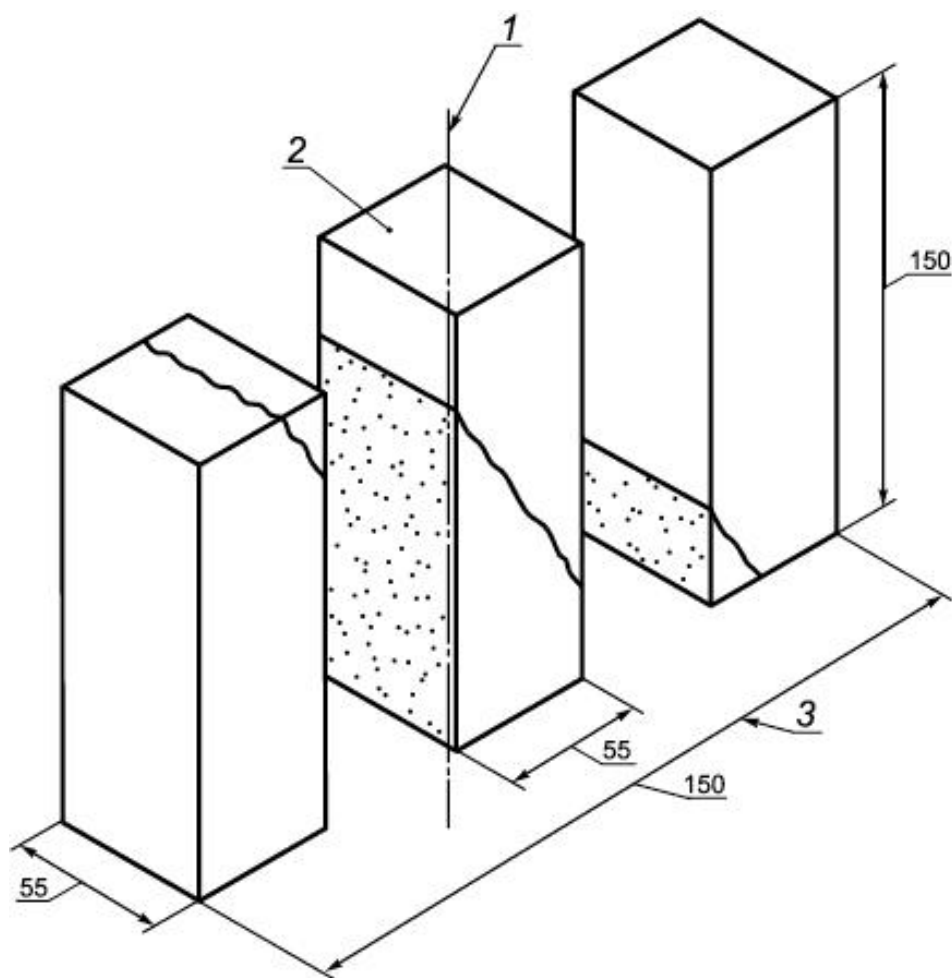
Рисунок К.3 - Схема выпиливания контрольного образца-призмы
