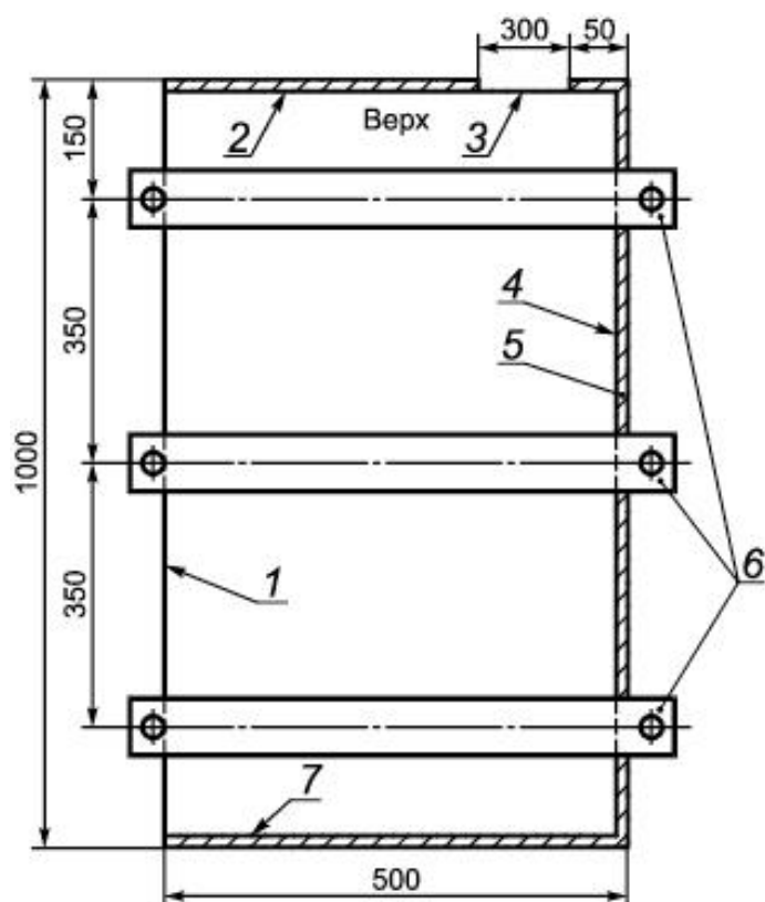
Рисунок Д.2 - Сборный образец-плита в кондукторе для формирования зазора - вид спереди
