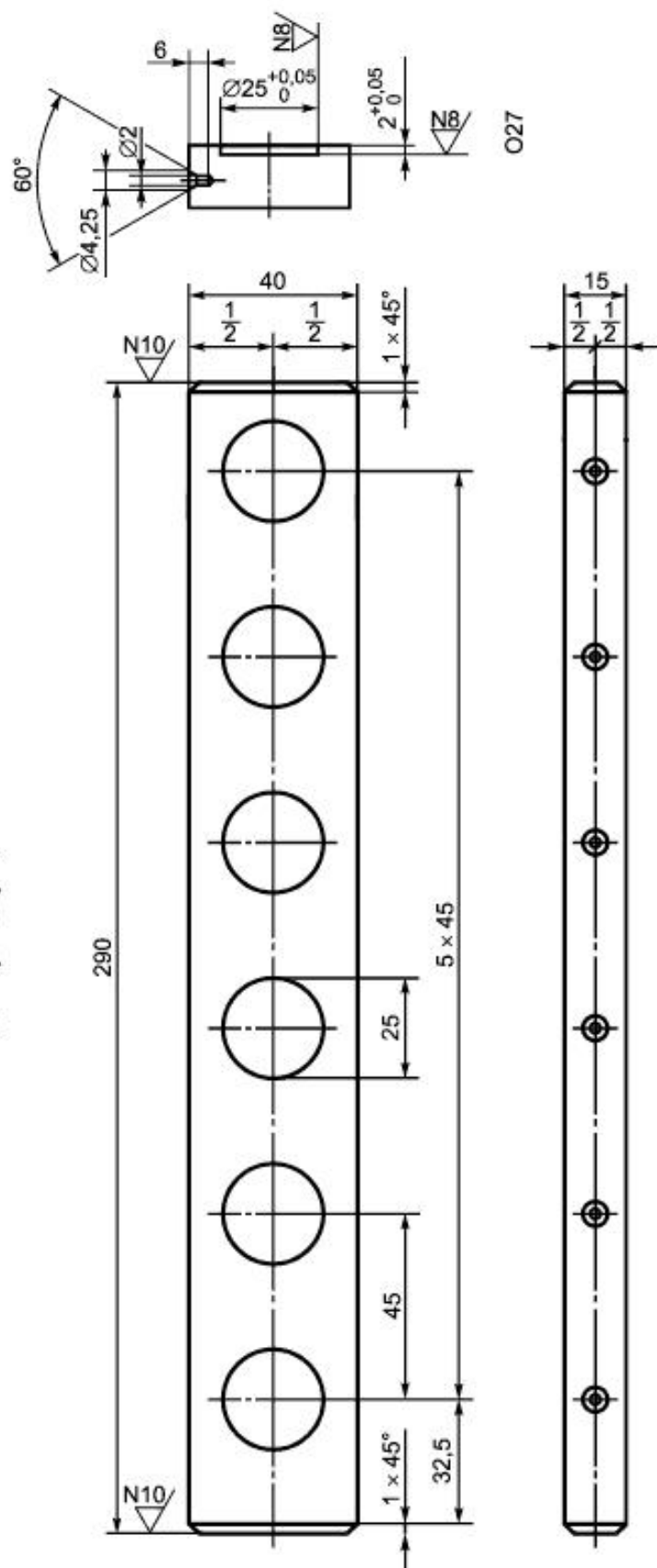
Рисунок М.1 - Модульная рейка
